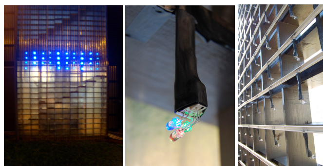
Fig. 1. Imagem do efeito dos LED's na grelha no protótipo construído. Fig. 2. Estrutura de fixação dos LED's RGB. Fig. 3. Estrutura dos LED's fixada na grelha de madeira do edifício.
